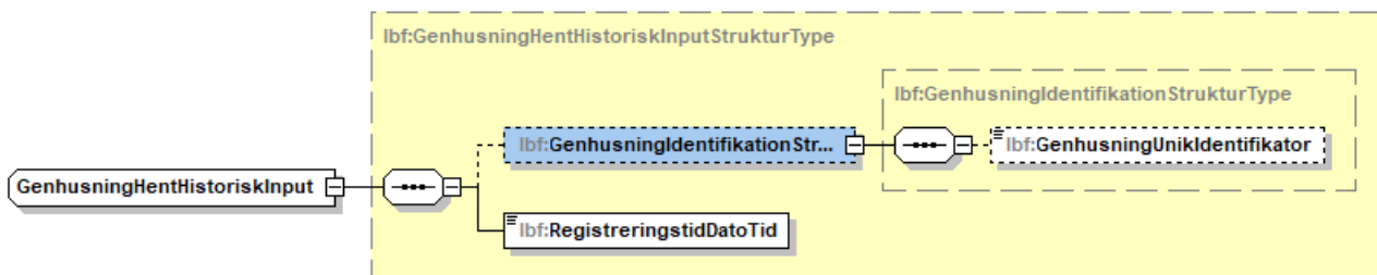
Figur 95 - Illustration af GenhusningHentHistoriskInputStruktur
