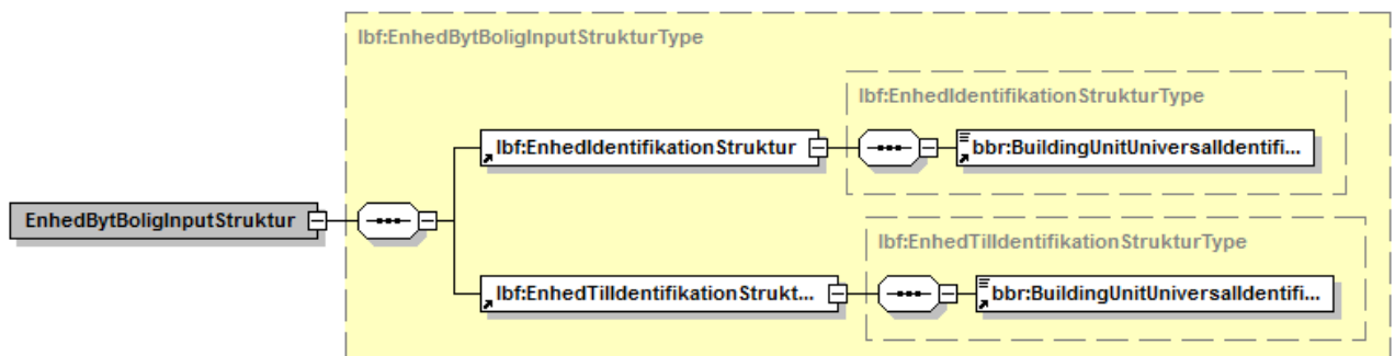
Figur 74 - Illustration af EnhedBytBolig
