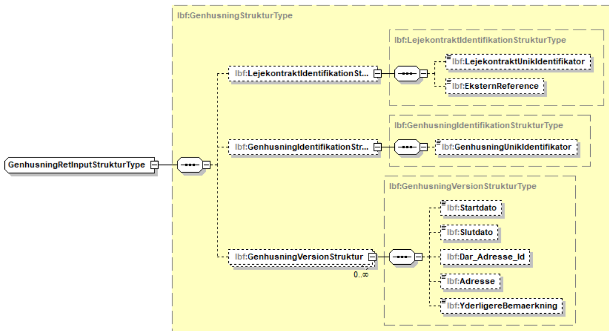
Figur 93 - Illustration af GenhusningRetInputStruktur
