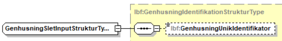
Figur 94 - Illustration af GenhusningSletInputStruktur
