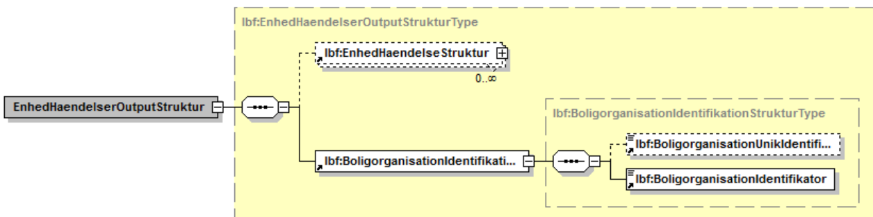
Figur 80 - Illustration af EnhedHaendelserOutputStruktur
