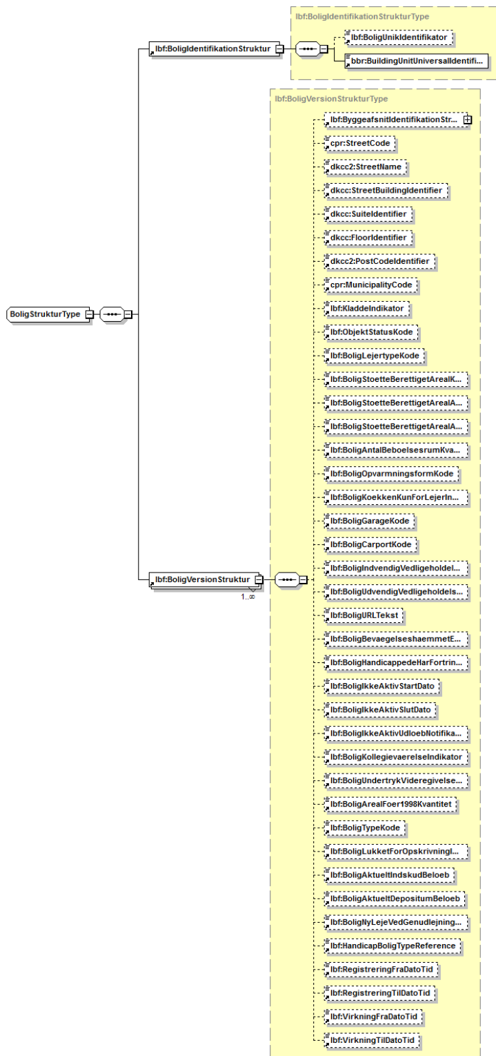
Figur 34 - Illustration af strukturen for en Bolig.
