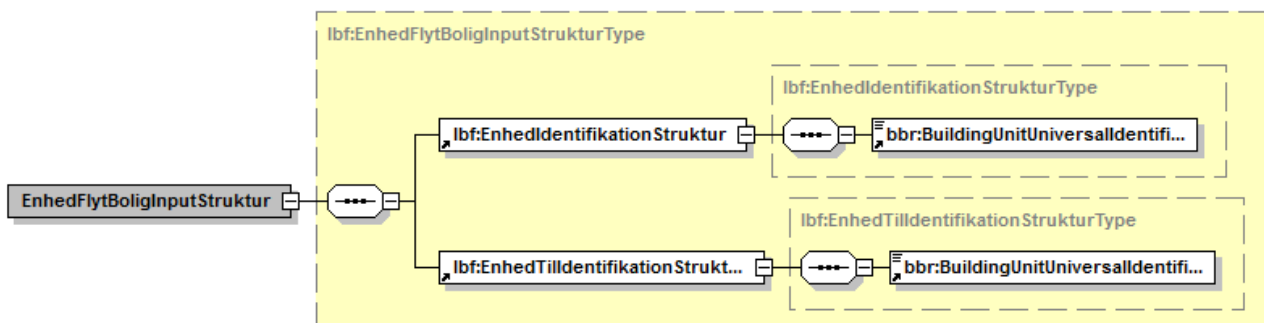
Figur 76 - Illustration af EnhedFlytBoligInputStruktur
